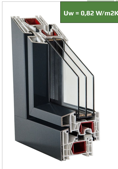
AluClipPro
